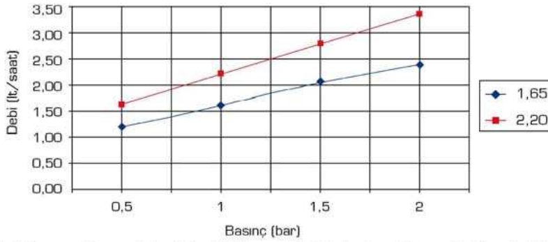
Basınç Debi İlişkisi
